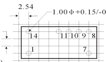
DIP 14 封装
